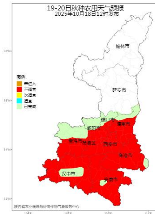
图 4 10 月 19-20 日秋种农用天气预报
