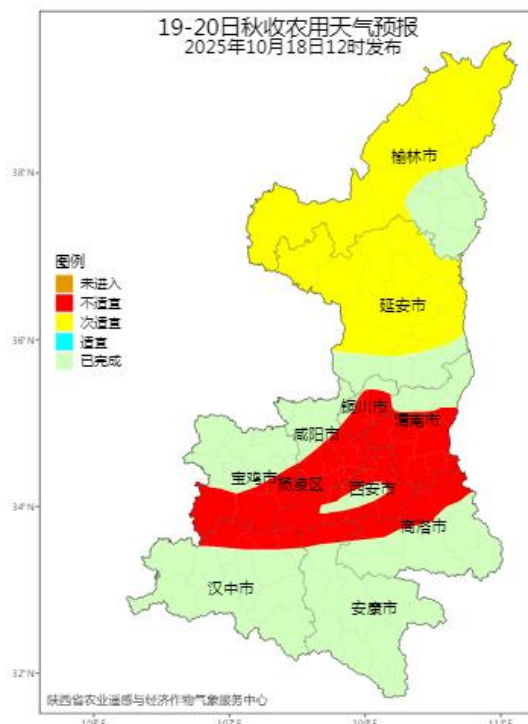
图 3 10 月 19-20 日秋收农用天气预报
