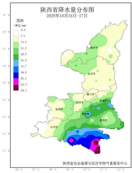
图 1 16-17 日降水量分布
