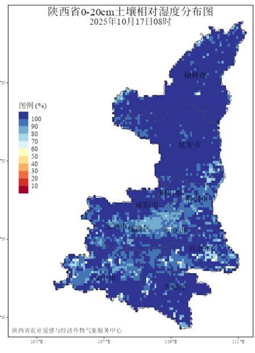
图 2 17 日 08 时土壤相对湿度
